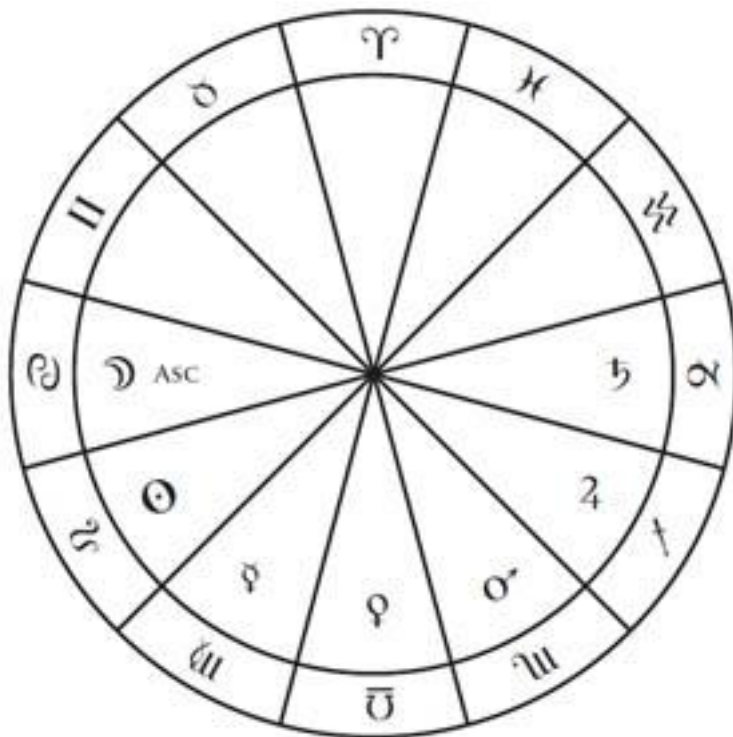
Εικ. 4 - Χάρτης Thema Mundi – πηγή: Wikipedia
