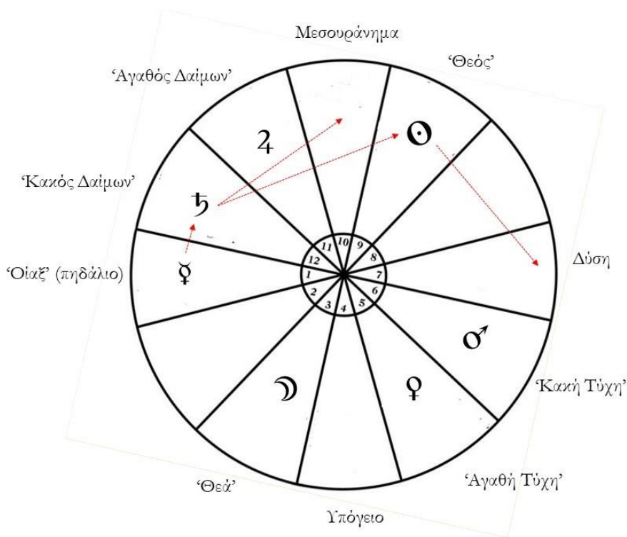
Εικ.2 –Το σχήμα της χαράς των πλανητών κατά την Ελληνιστική Αστρολογία
