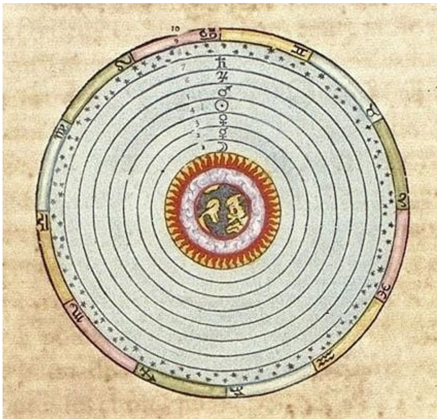
Εικ.1 – Το σύστημα του Πτολεμαίου – J. W. Blaeu, Geographia , Amsterdam, 1667, Firenze Museo di Storia della Scienza.
